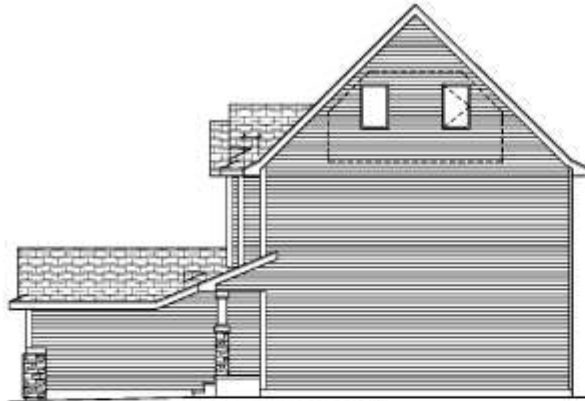
RIGHT ELEVATION "A"
